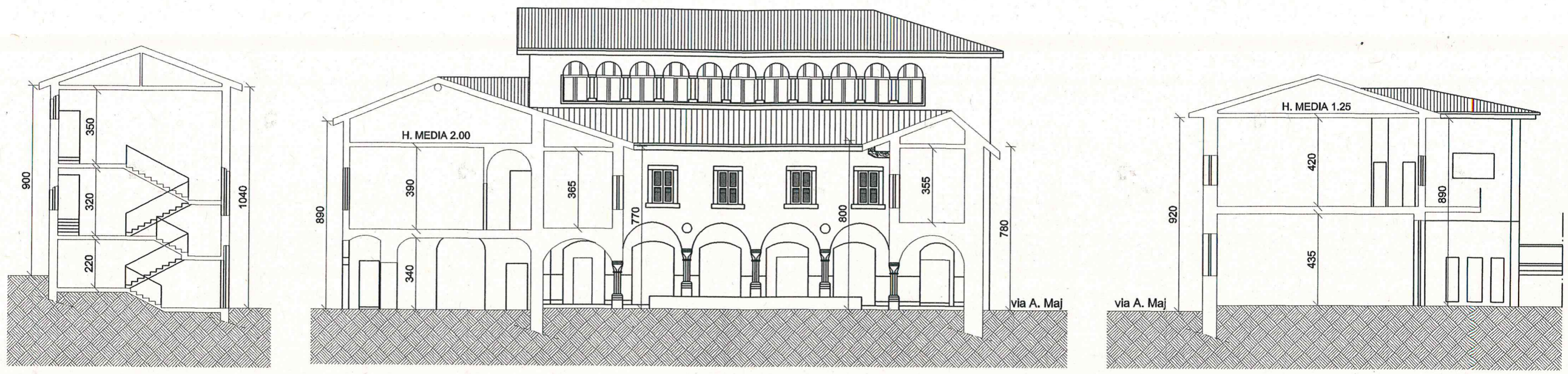
SEZIONE B-B
